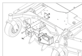
Kit zavorra anteriore Peso rimovibile per migliorare l'equilibrio della macchina durante il lavoro in pendenza.
