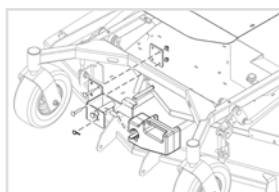
Sada předního závaží Odnímatelné závaží pro zlepšení vyvážení stroje při práci ve svahu.
